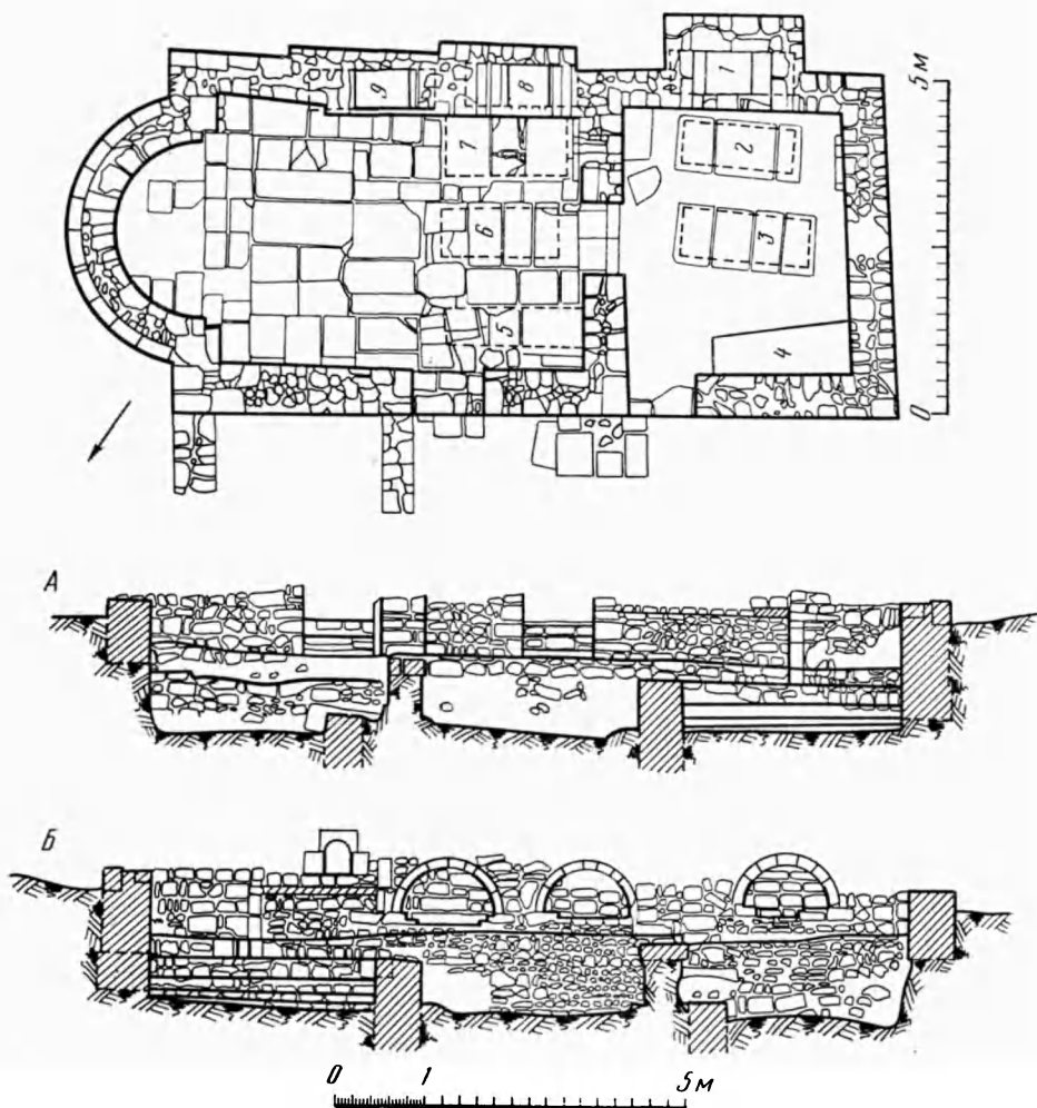
Рис. 2. Храм. План и разрезы; 1—9 — могилы.
